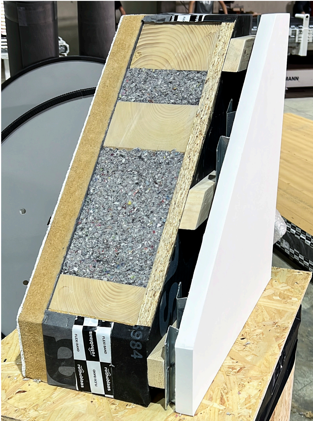
FIG. 10 SISTEMA WOODFRAME
